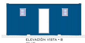
ELEVACIÓN VISTA - B
